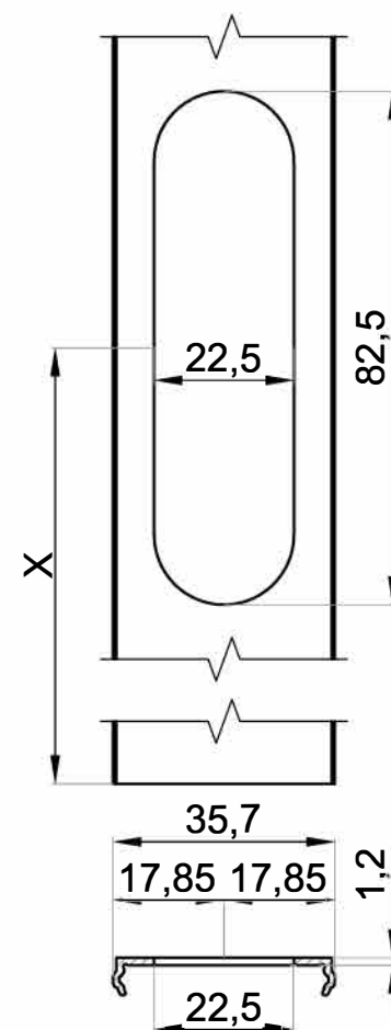
Frézování- PF-M
